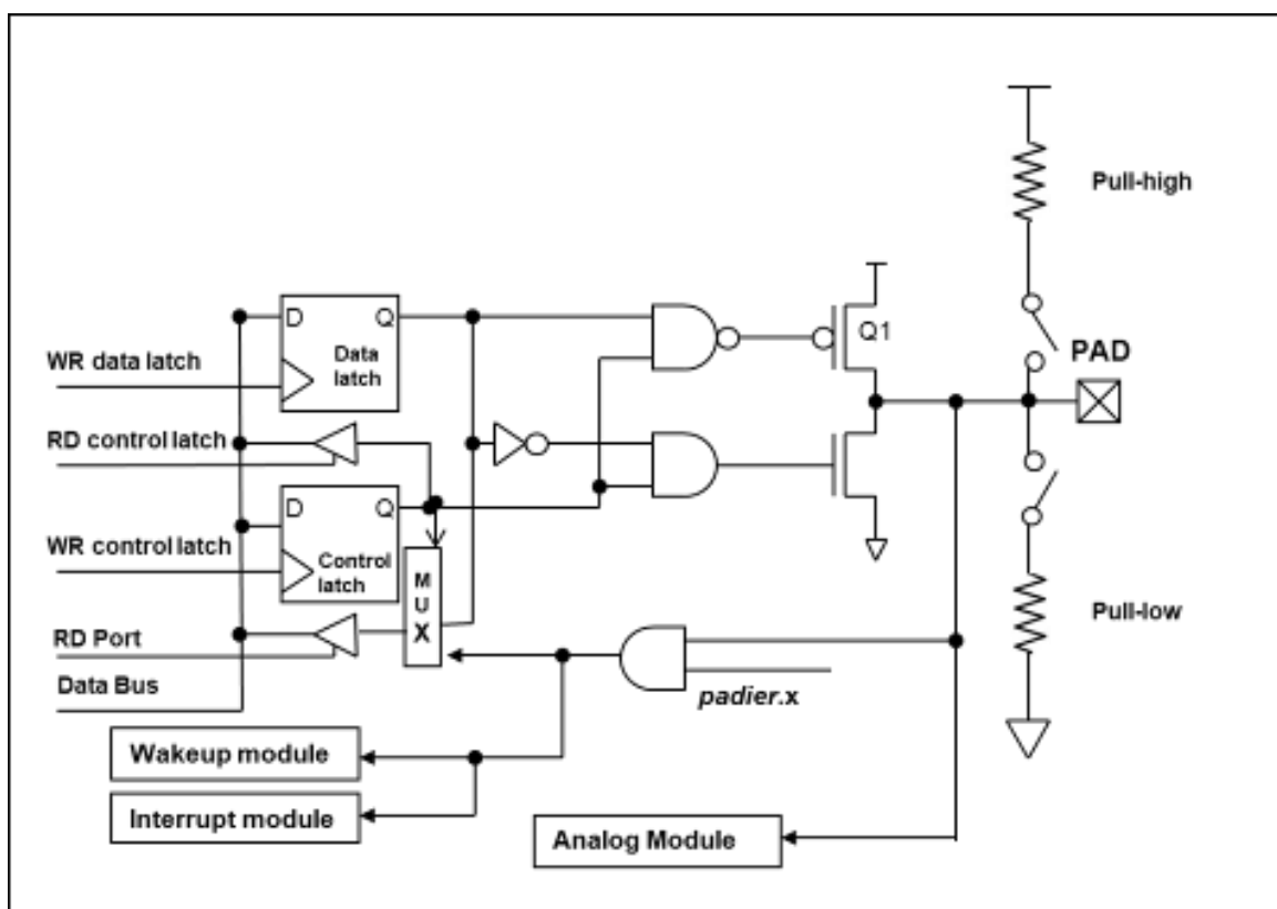
图 12: IO 引脚缓冲区硬件图
