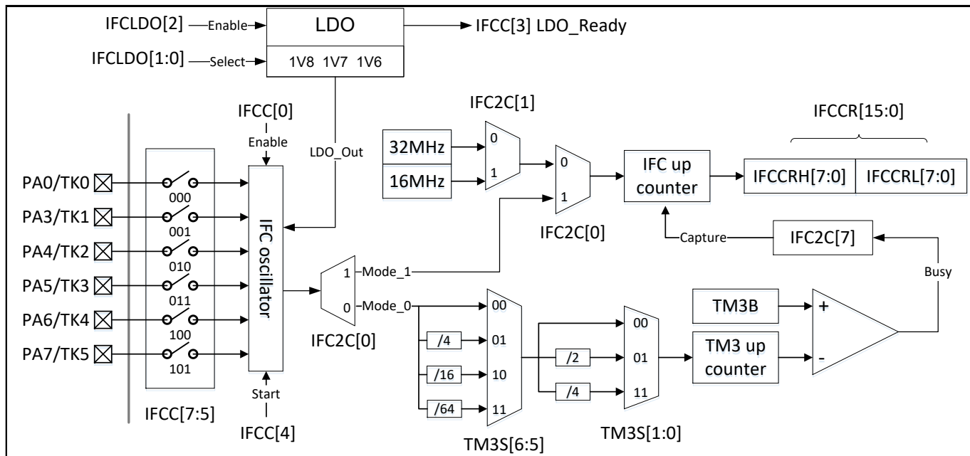
图 23: 触摸检测电路的功能方框图
