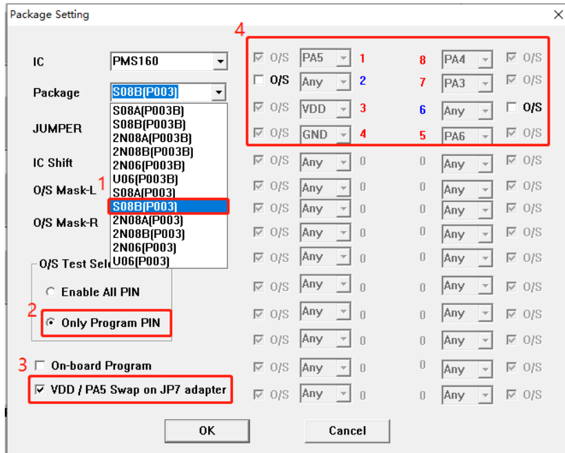
图 26: PMS160-S08B 在 P003 转档配置
