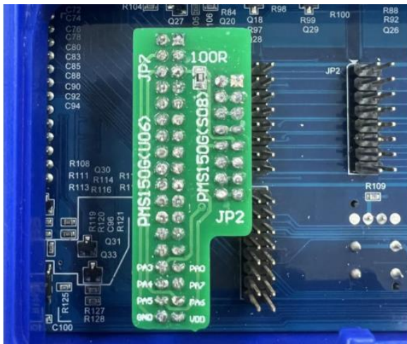
图 14: JP7 连接实物图
