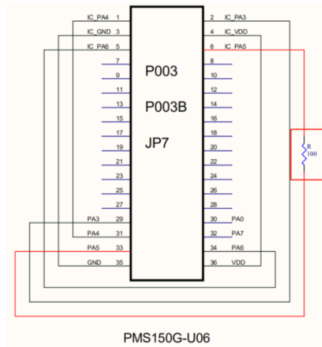
图 16: JP7 连接原理图
