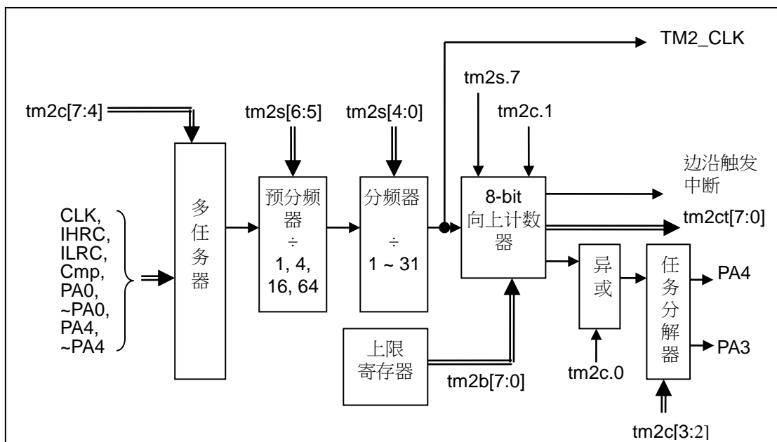
图 9: Timer2 模块框图
