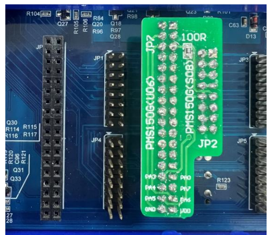
图 15: JP2 连接实物图
