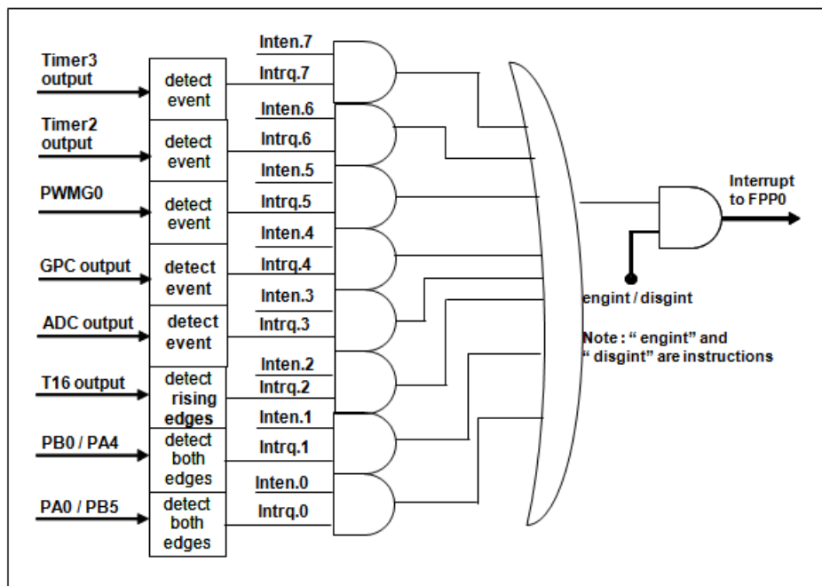
图 19: 中断控制器硬件框图
