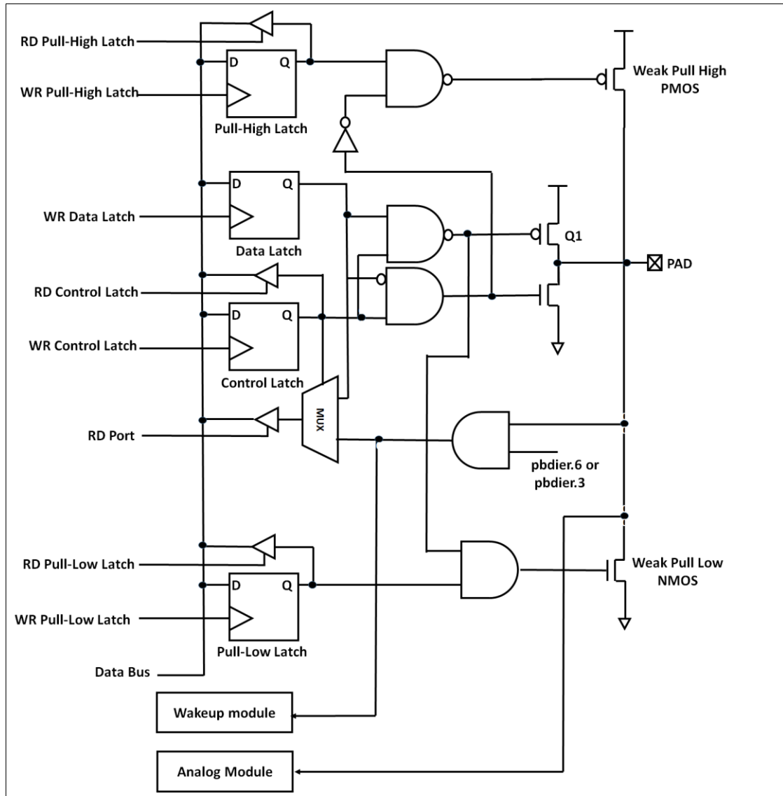
图 20: IO 引脚缓冲区硬件图
