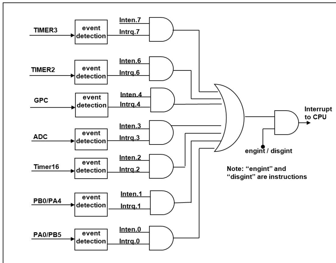
图 17：中断控制器硬件框图
