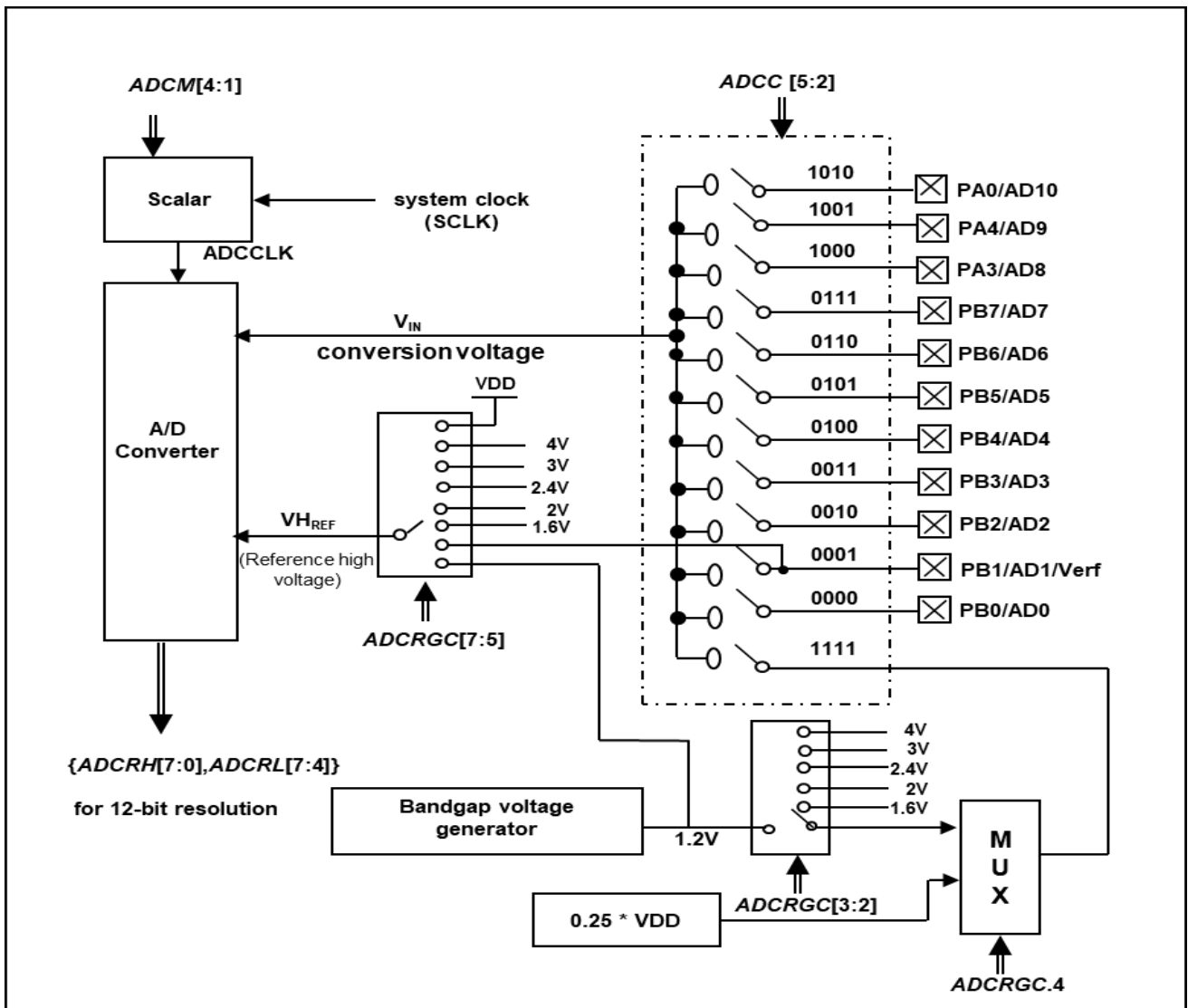
图 19: ADC 模块框图
