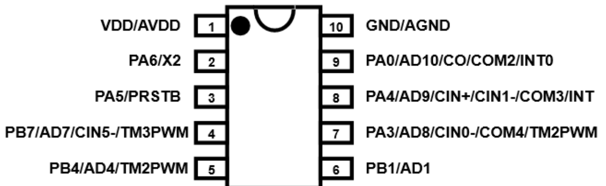
PFS122B-M10 (MSOP10-118mil)
