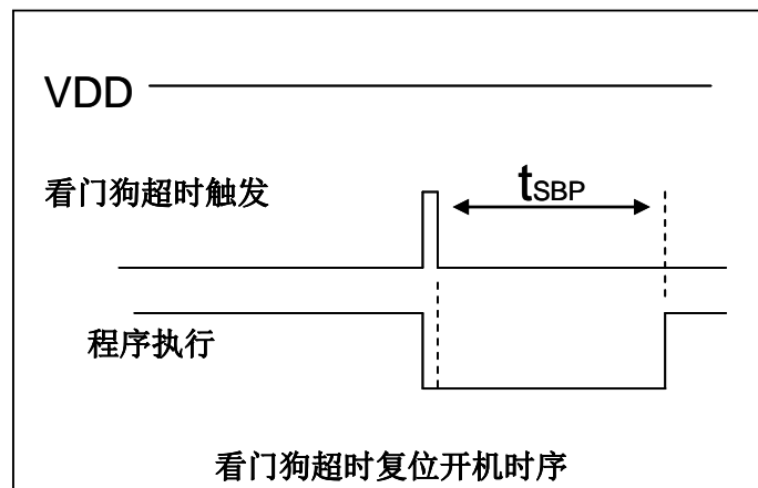
图 16：看门狗超时溢出时序图
