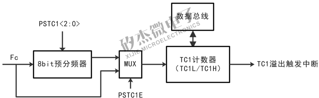
TC1 结构框图
