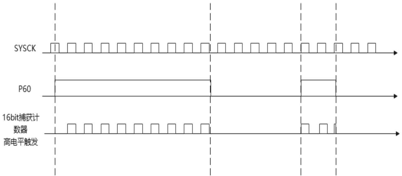
16bit捕获计数器由低八位的TBRE和高八位的TCO组成
