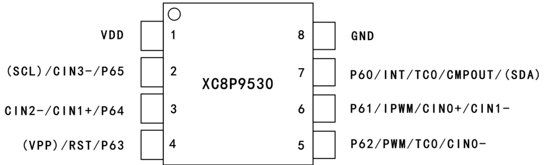
XC8P9530-8PIN 脚位图
