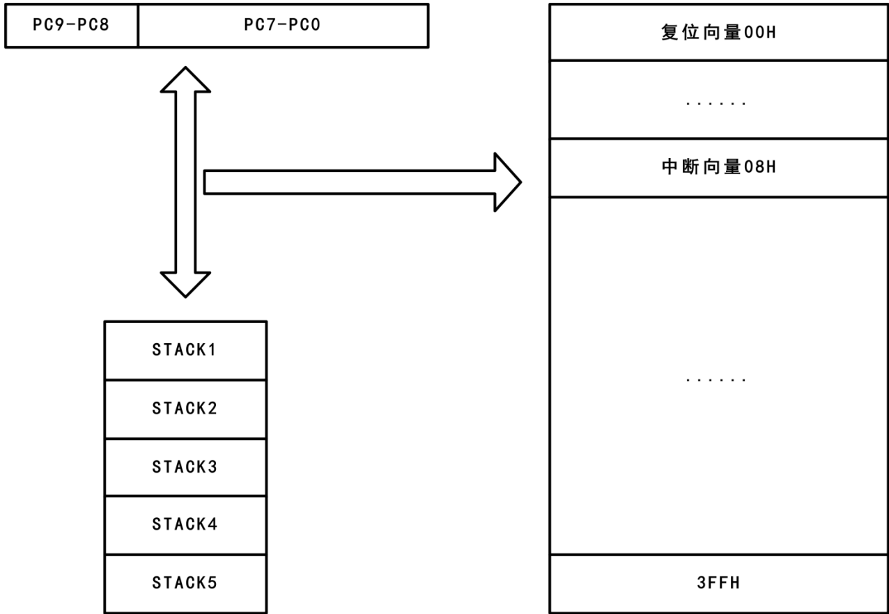
程序存储区结构图
