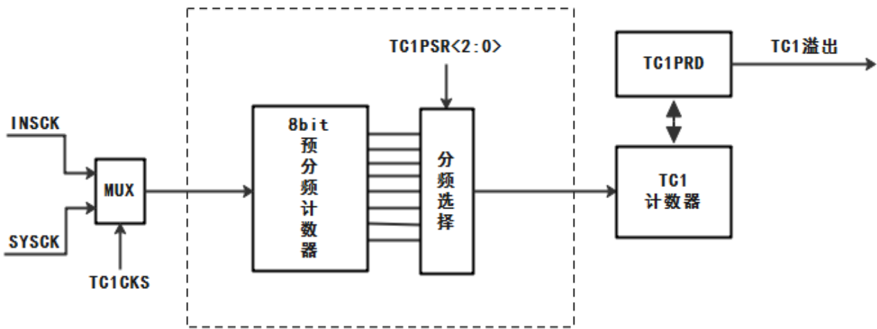
TC1 结构框图
